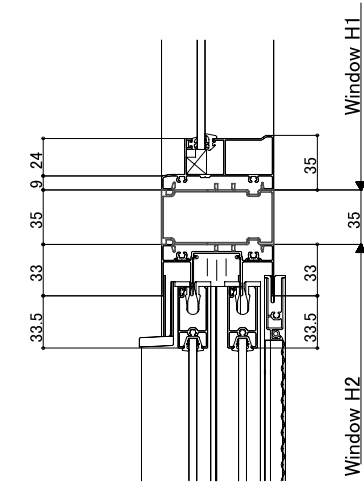
<Transom>
