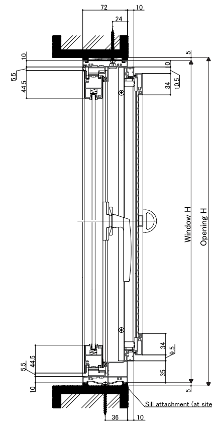
<Vertical section: Casement with scr een>
