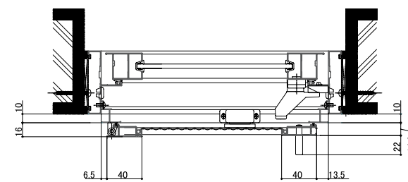
<Horizontal section: Casement with scr een>
