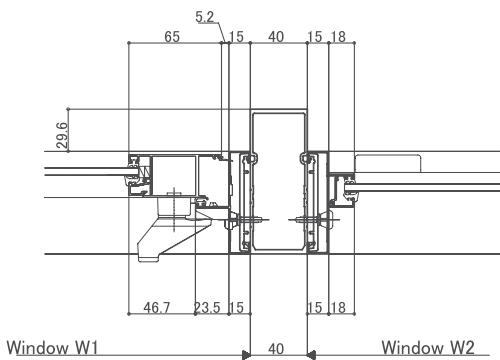
<Mullion (medium)>
