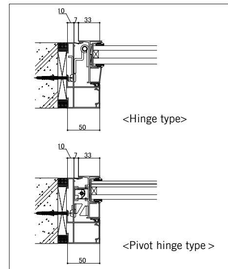
<Jamb detail>
